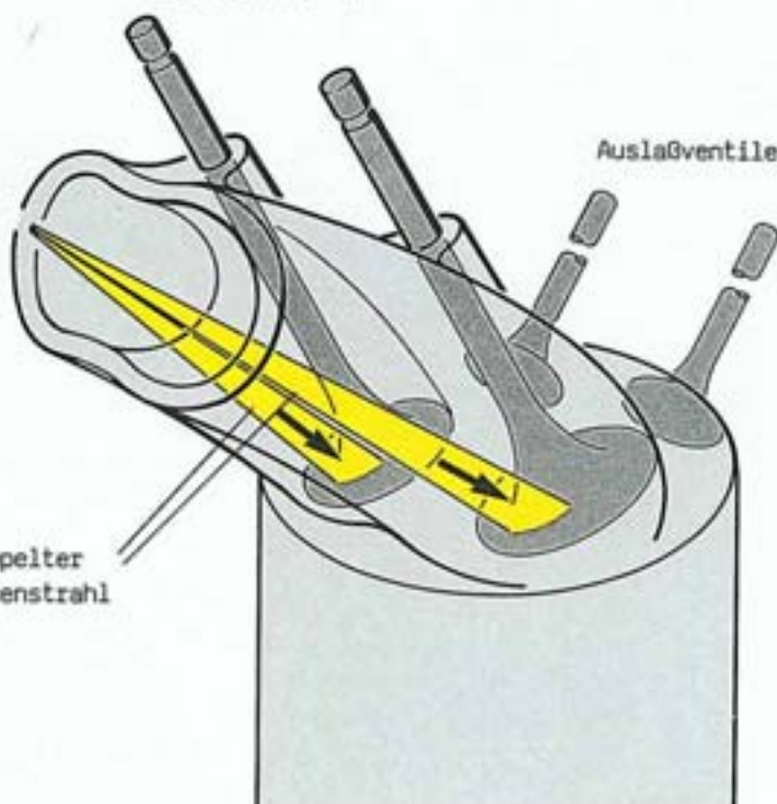
Einlaßventile
